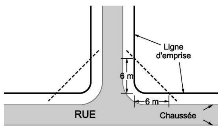
Croquis 9.1 Aménagement d'un triangle de visibilité
